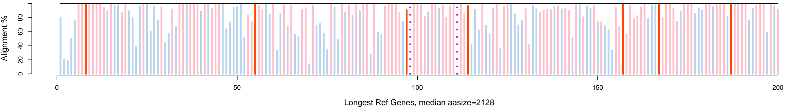
Gene set: dapplx10evg (85% ref align, 56% best)
