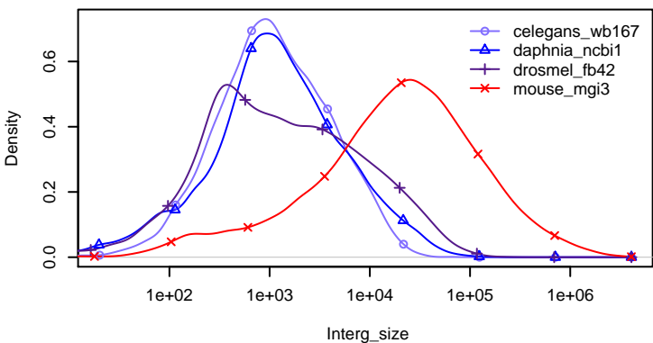
Eukaryote Interg_size
